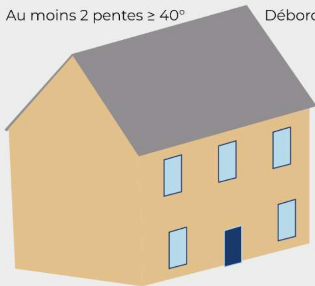
Toiture à deux pans
